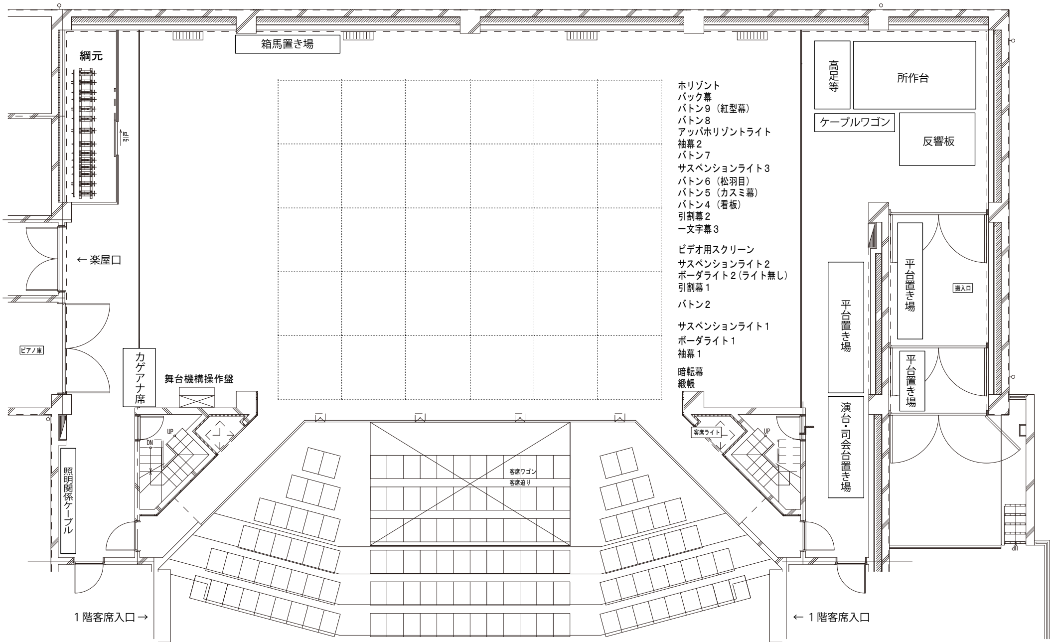
宜野座文化センター(がらまんホール) 舞台平面図
